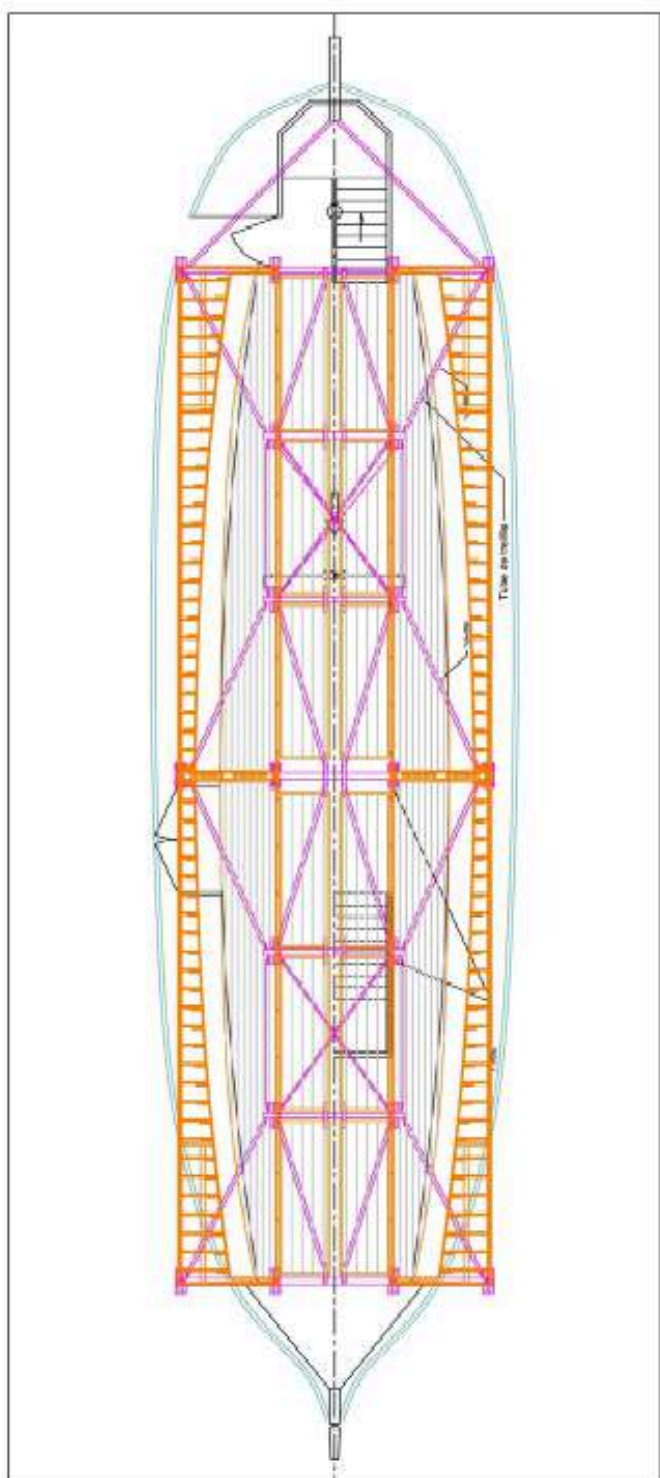
Disposition générale de la structure (en orange les 4 conteneurs / en magenta le marbre)
